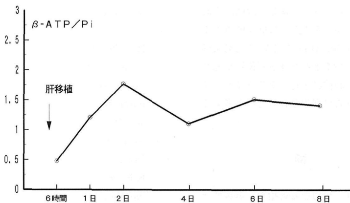
図21 肝移植後の \beta -ATP/Pi の経時的変化
