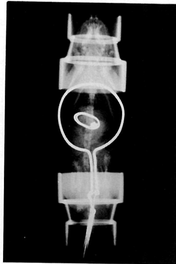
図5 31 P-MRS 測定時のラットのX線写真 レーザーコーイルはサーフェスコイルが中心となるように設置する。実際の測定にはオシロスコープを使用して位置を決定する。
