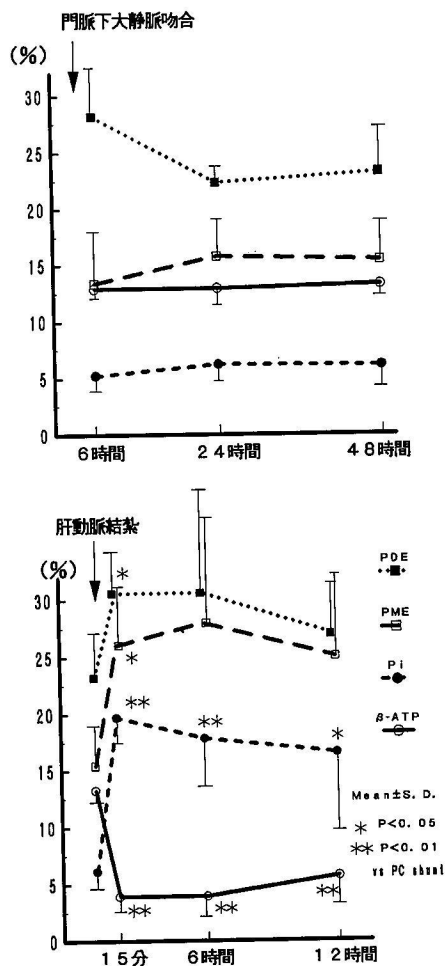
図12 各成分の経時的変化 (虚血肝障害モデル群) 上図は門脈一下大静脈吻合後6時間から48時間の変化。
